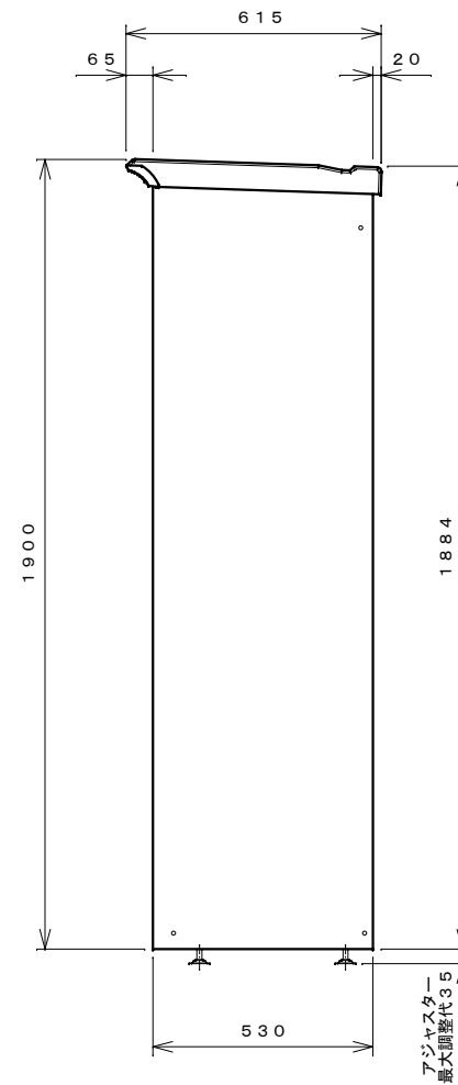
右側面図
