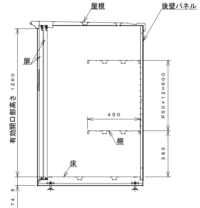
側面断面図
