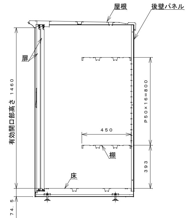
側面断面図
