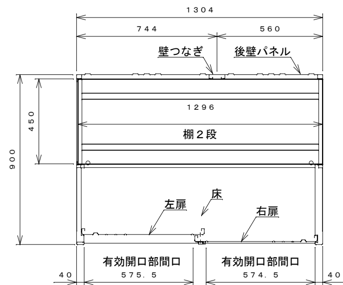
平面断面図
