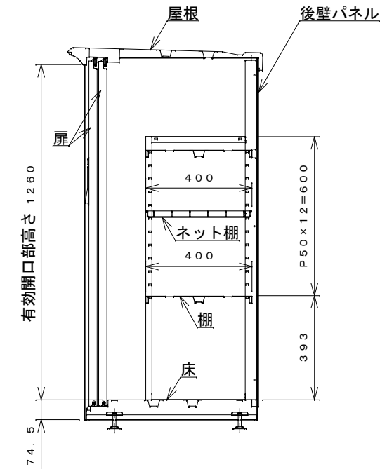
側面断面図
