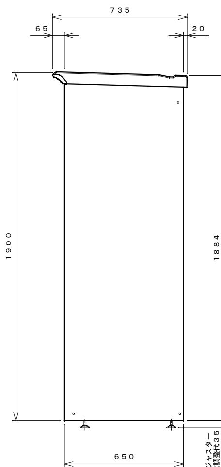
右側面図
