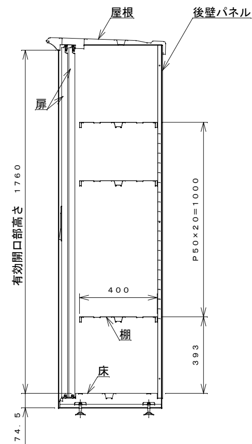
側面断面図
