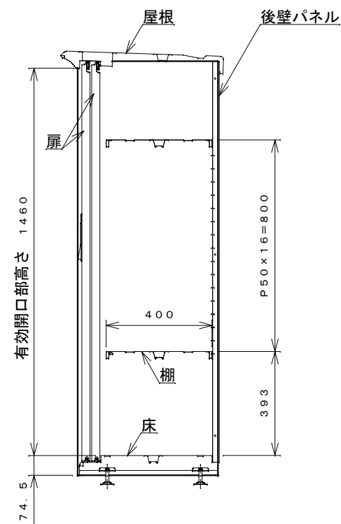
側面断面図
