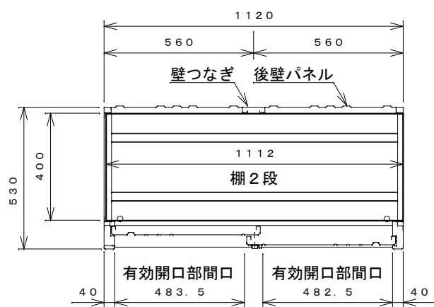
平面断面図
