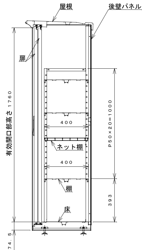
側面断面図
