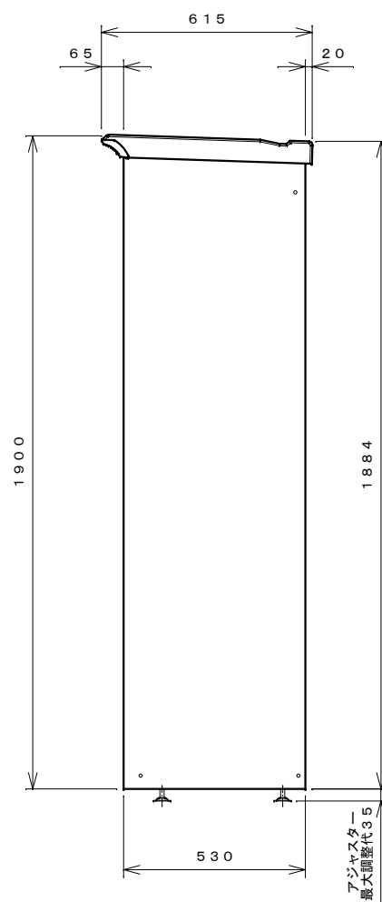
右側面図
