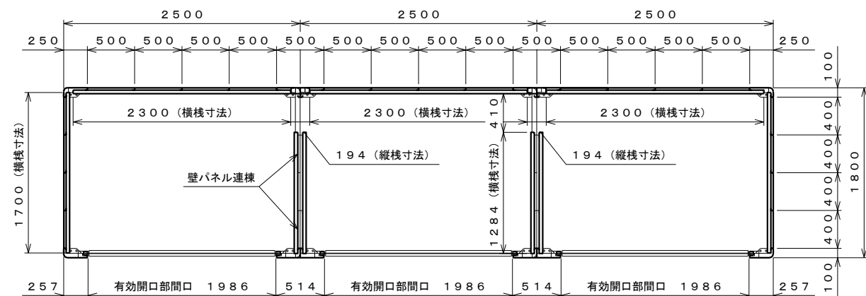
平面図 S=1:40
