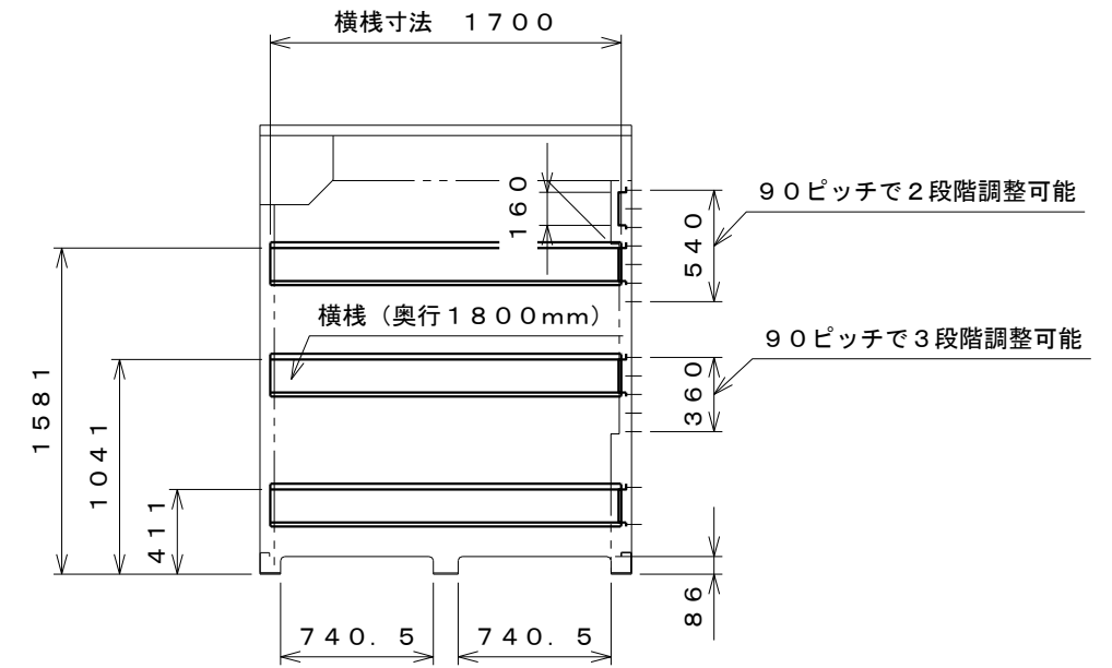
内面図 S=1:40
