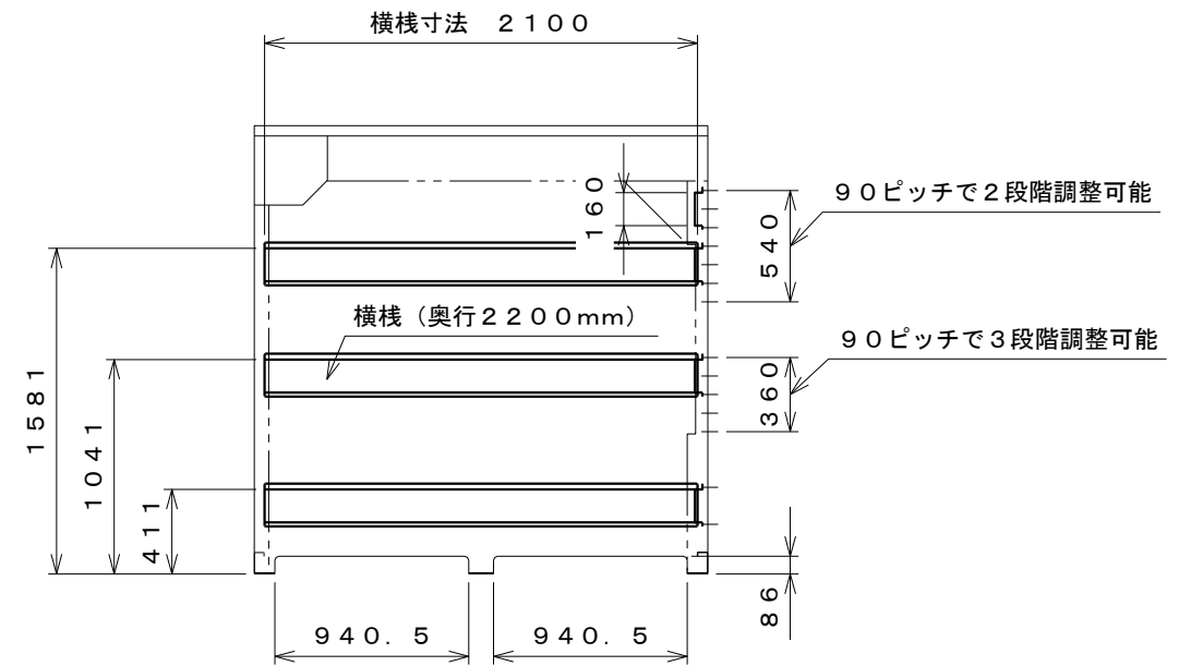
内面図 S=1:40
