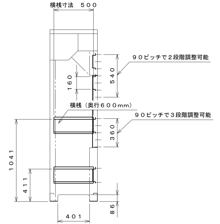
内面図 S=1:25
