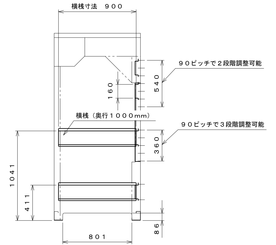
内面図 S=1:25
