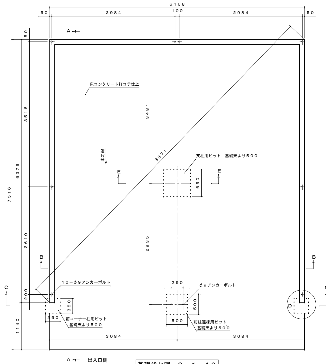
基礎伏せ図 S=1:40
