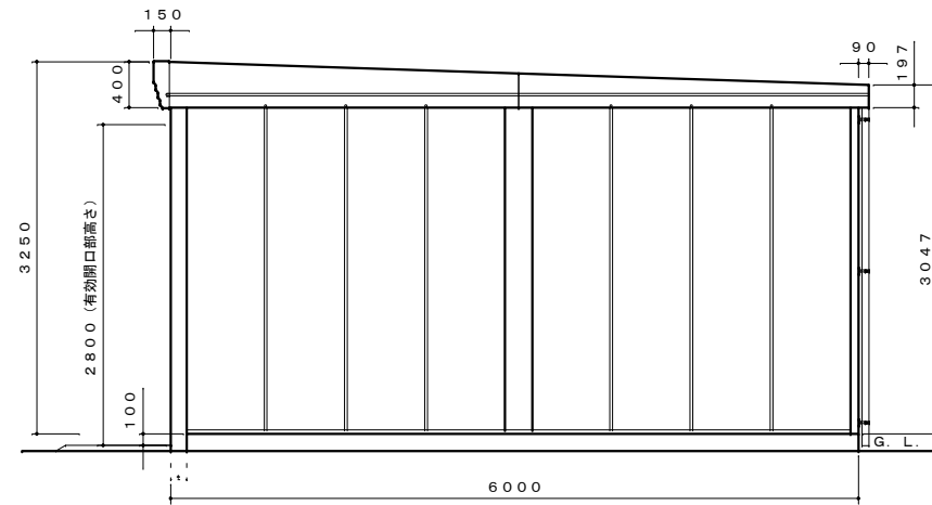
側面図 S=1:50
