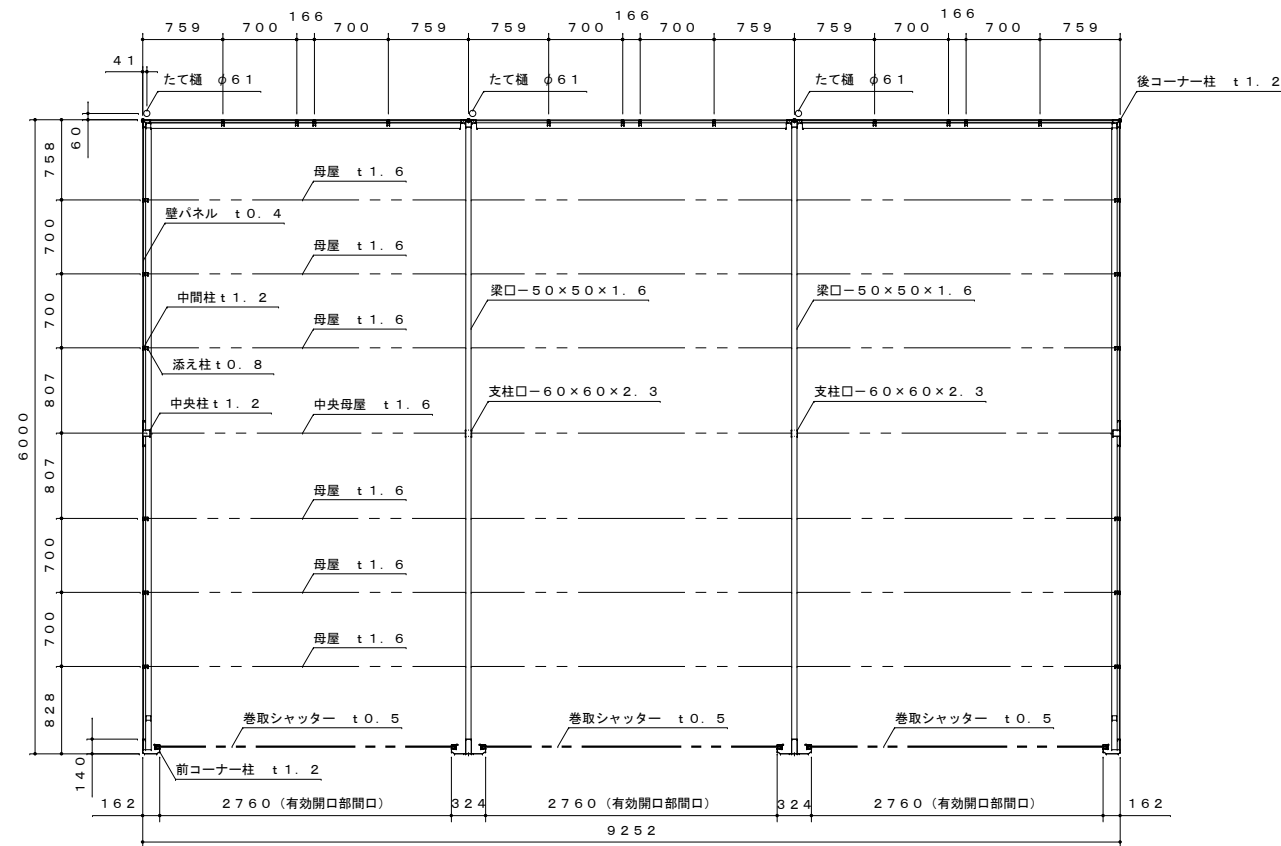
平面図 S=1:50
