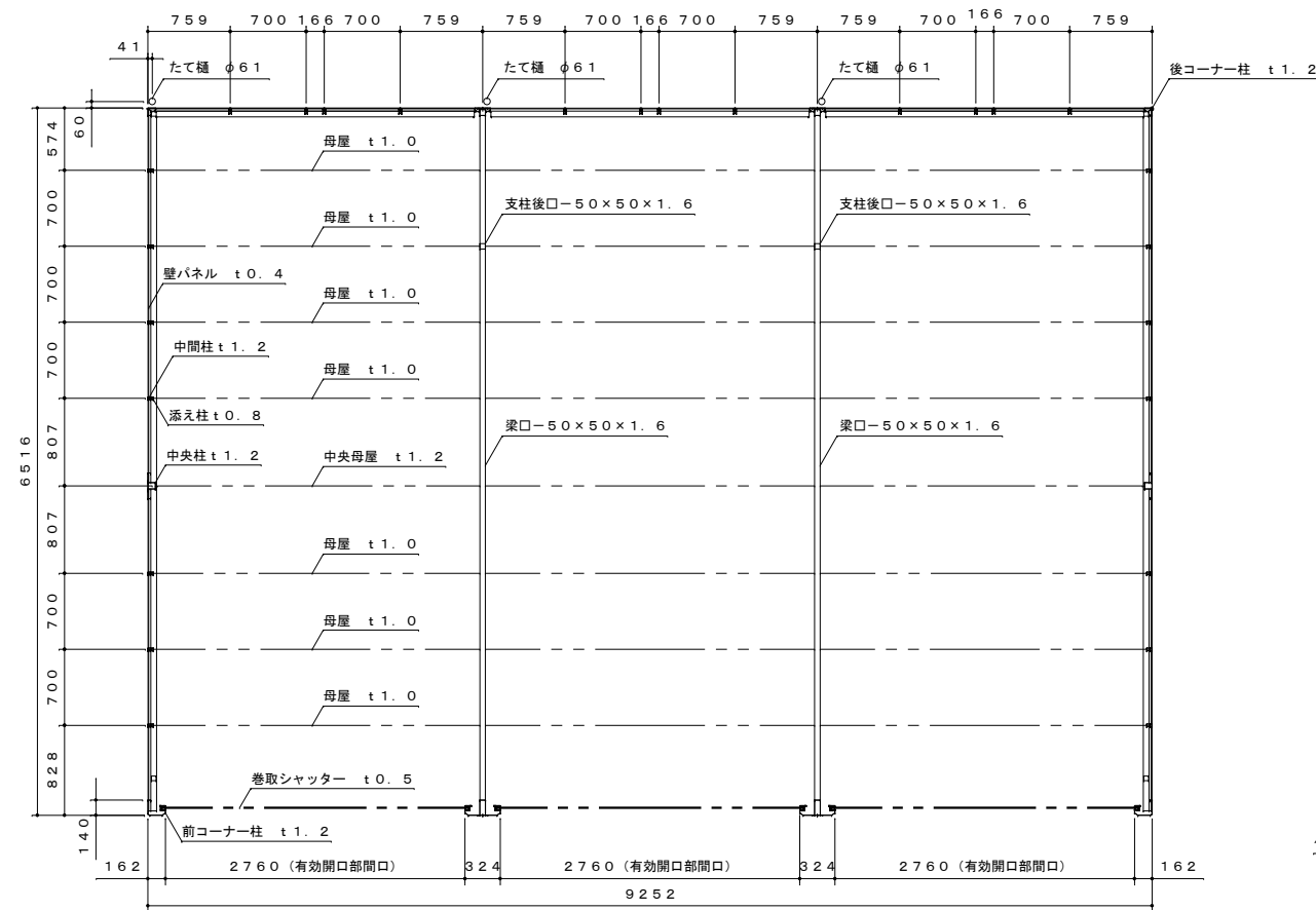
平面図 S=1:50
