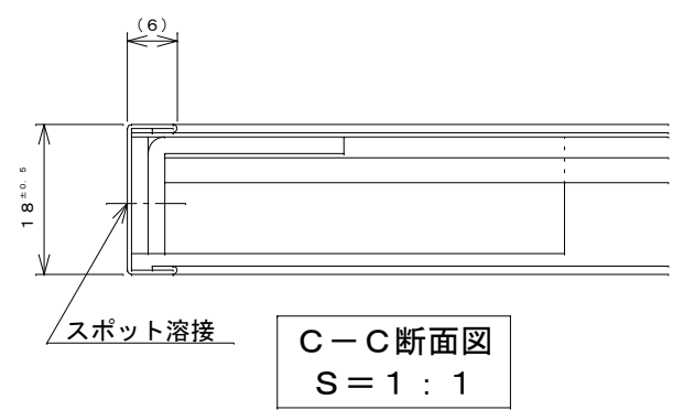
D部詳細図 S=1:1
