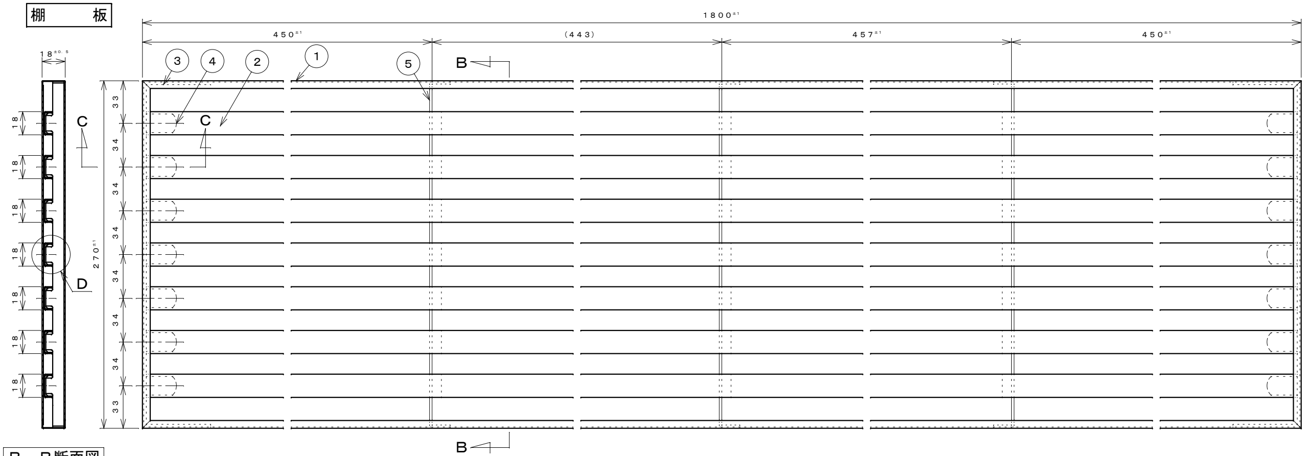
B-B断面図
