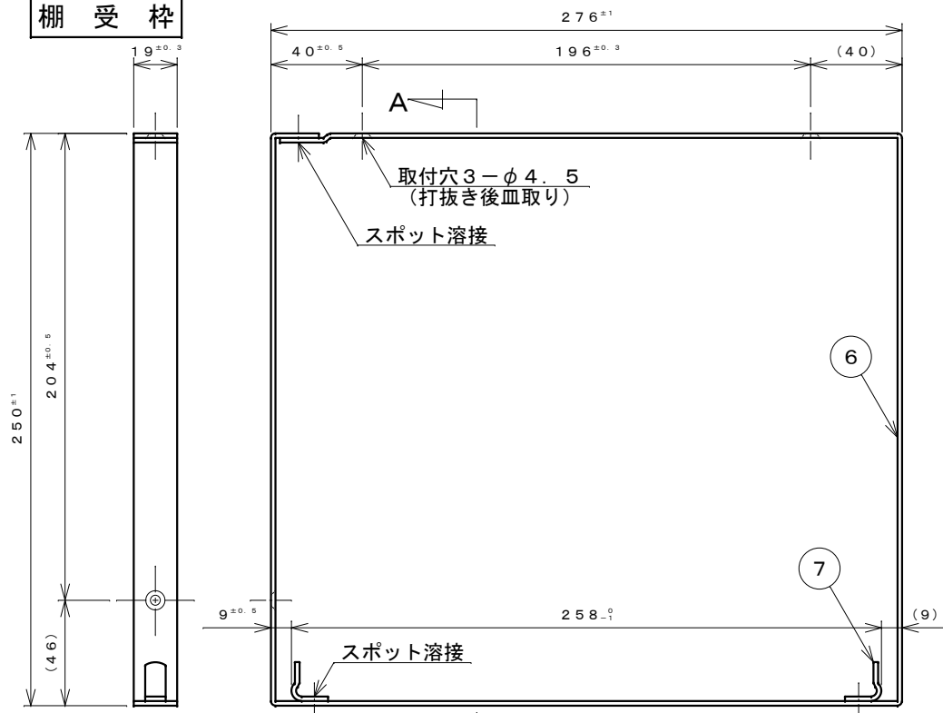
A-A断面図
