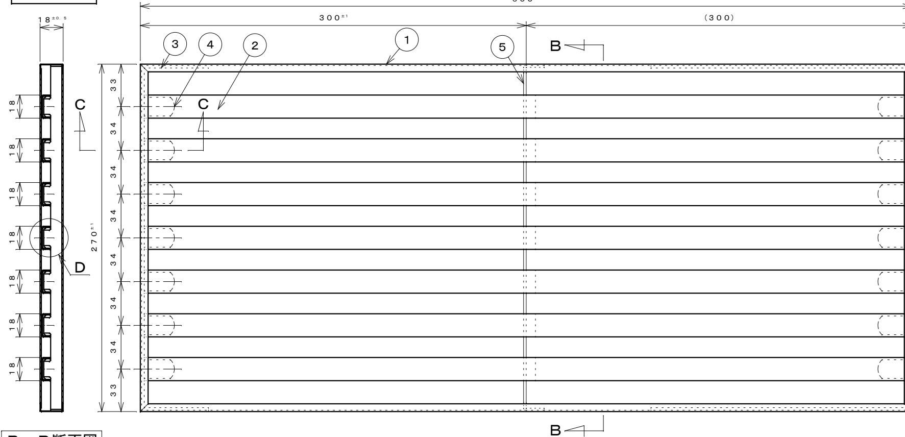
B-B断面図
