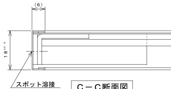
C-C断面図 S=1:1
