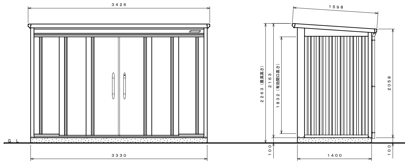
正面図 S=1:30
