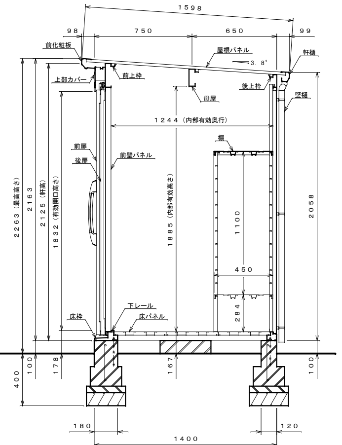
側面断面図 S=1:20
