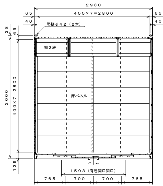
平面図 S=1:40
