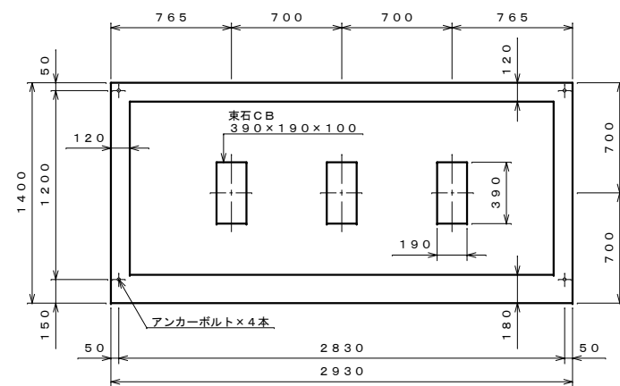
基礎伏せ図 S=1:30
