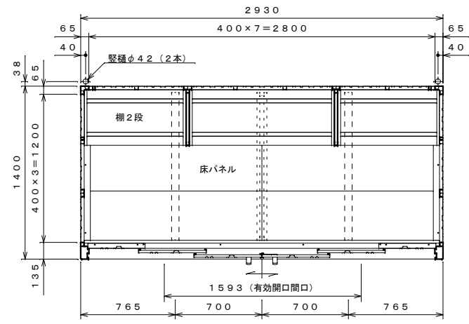
平面図 S=1:30
